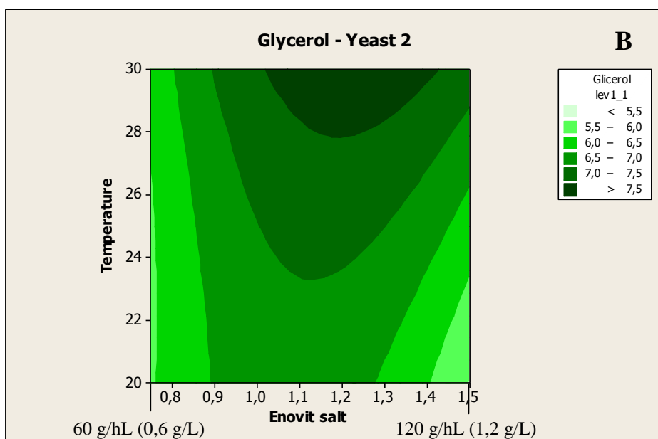
Figura 10 – Representação da interacção entre os diversos níveis de temperatura e da massa de nutrientes (sais Enovit) por 1,25 L, na produção de glicerol para a levedura Saccharomyces cerevisiae Fermol ® Reims Champagne (Pascal Biotech ® ) (A) e Saccharomyces cerevisiae ICV ® D47 (B).
