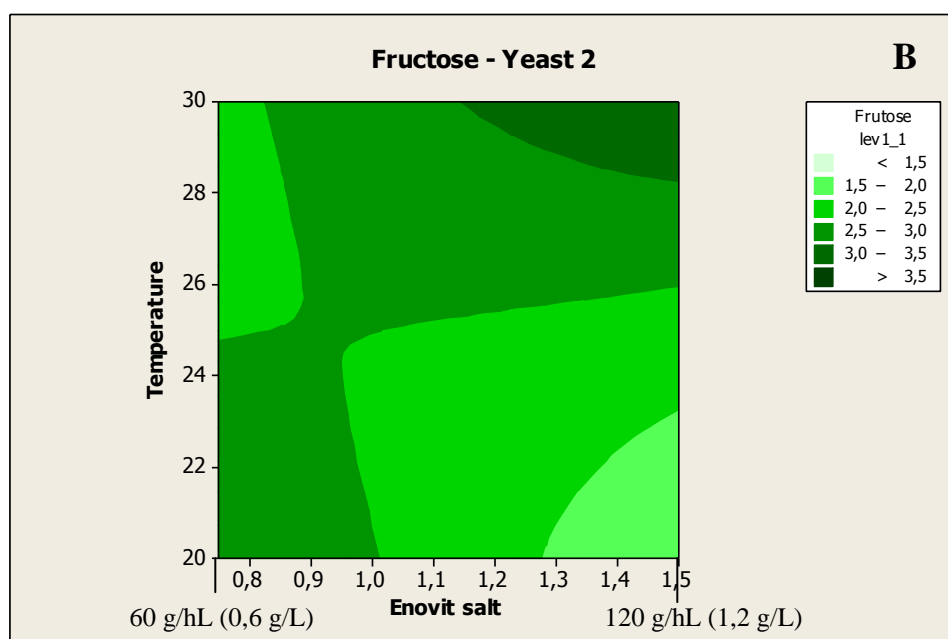
Figura 12 – Representação da interacção entre os diversos níveis de temperatura e da massa de nutrientes (sais Enovit) por 1,25 L, na concentração final de frutose para a levedura Saccharomyces cerevisiae Fermol ® Reims Champagne (Pascal Biotech ® ) (A) e Saccharomyces cerevisiae ICV ® D47 (B).
