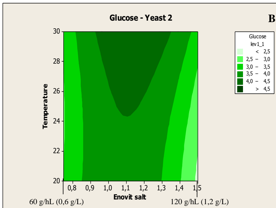
Figura 11 – Representação da interação entre os diversos níveis de temperatura e da massa de nutrientes (sais Enovit) por 1,25 L, na concentração final de glucose para a levedura Saccharomyces cerevisiae Fermol ® Reims Champagne (Pascal Biotech ® ) (A) e Saccharomyces cerevisiae ICV ® D47 (B).
