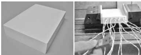
Fig. 1 Material compósito e instalação de termopares tipo K
