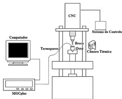
Fig. 2 Setup experimental para a furação dos blocos
