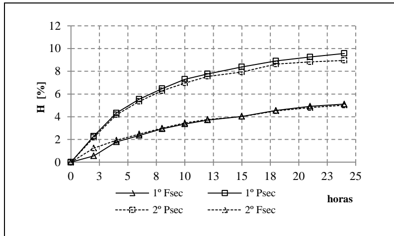
Figura 7: Teor em água para as madeiras de Pinho e de Freixo
