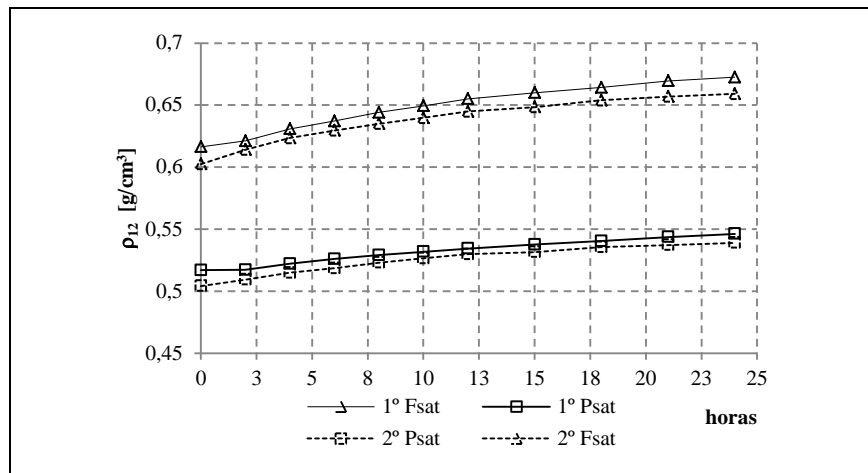
Figura 8: Massa volúmica de referência dos provetes secos e saturados
