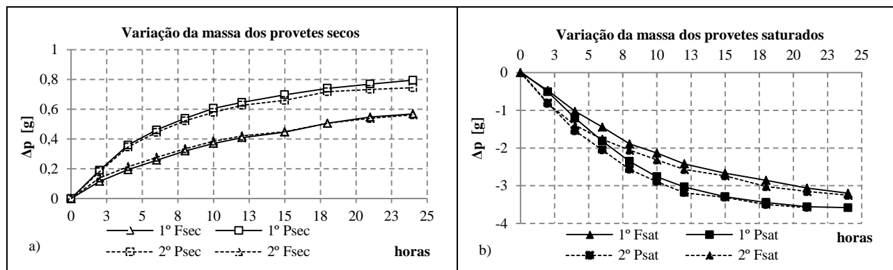
Figura 6: Variação da massa em provetes secos e em provetes saturados
