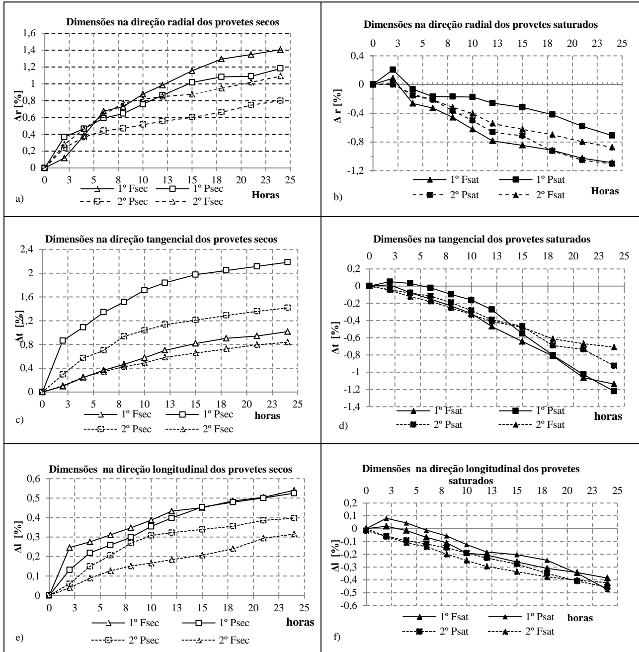
Figura 5: Variação dimensional dos provetes secos e dos provetes saturados
