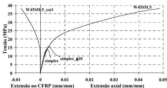
Figura 5 - Tensão versus extensão axial e extensão no CFRP nas séries do grupo C16S300 \phi 10
