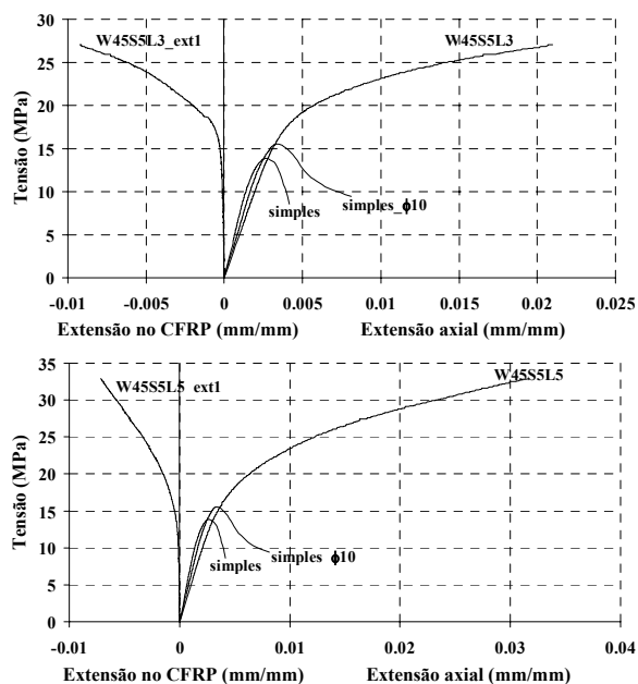
Figura 3 - Tensão versus extensão axial e extensão
