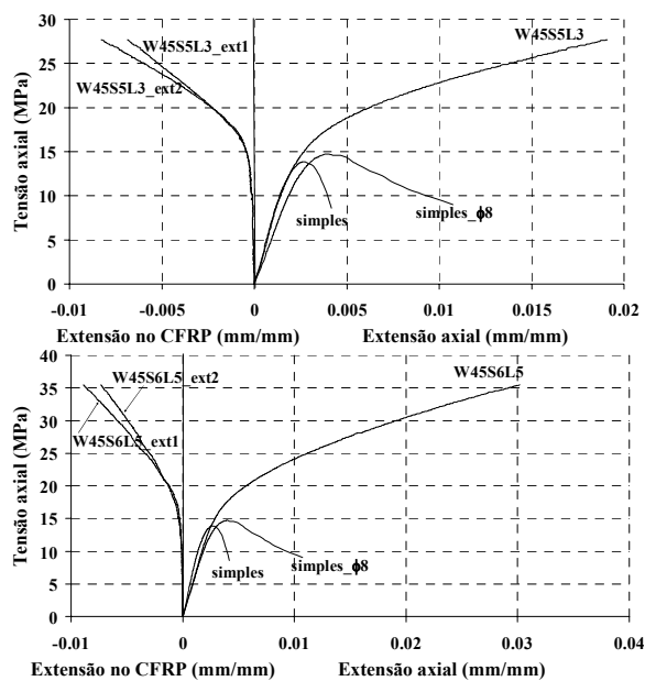
Figura 2 – Tensão versus extensão axial e extensão no CFRP nas séries do grupo C16S200 \phi 8
