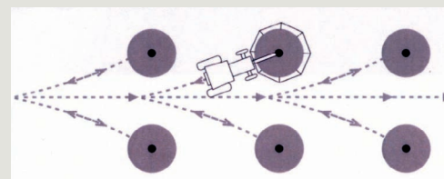
Figura 12 – Sistema II: trajetória do equipamento em solos planos ou pouco inclinados
