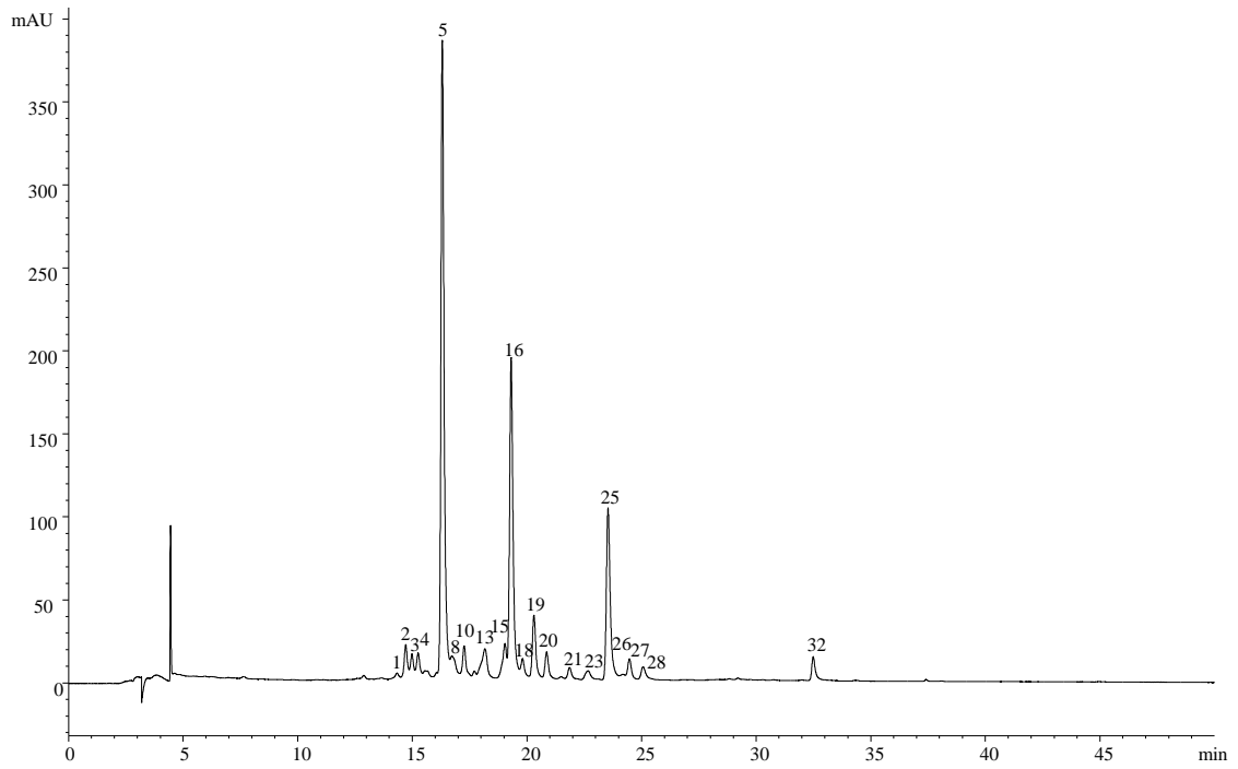
Figura 17. Perfil individual da composição fenólica na amostra PA1, registrado a 370 nm.
