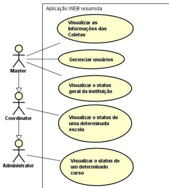
Figura 8: Diagrama de caso de uso da aplicação Web resumida.
