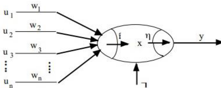
Figura 2: Neurônio artificial (reproduzido de Barreto [15])
