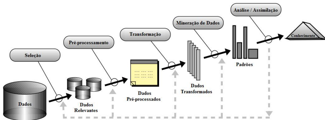
Figura 3: Etapas do processamento da mineração de dados (adaptado de Sharma et al. [20]).
