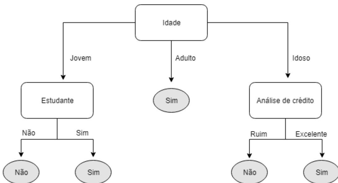
Figura 1: Exemplo de uma árvore de decisão (adaptado de Han et al. [10])
