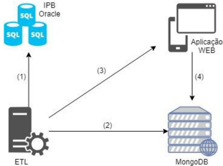
Figura 7: Diagrama da estrutura da ferramenta
