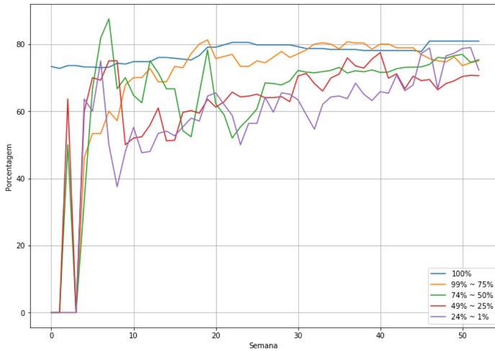
Figura 11: Recall por setores do atributo critical_rate
