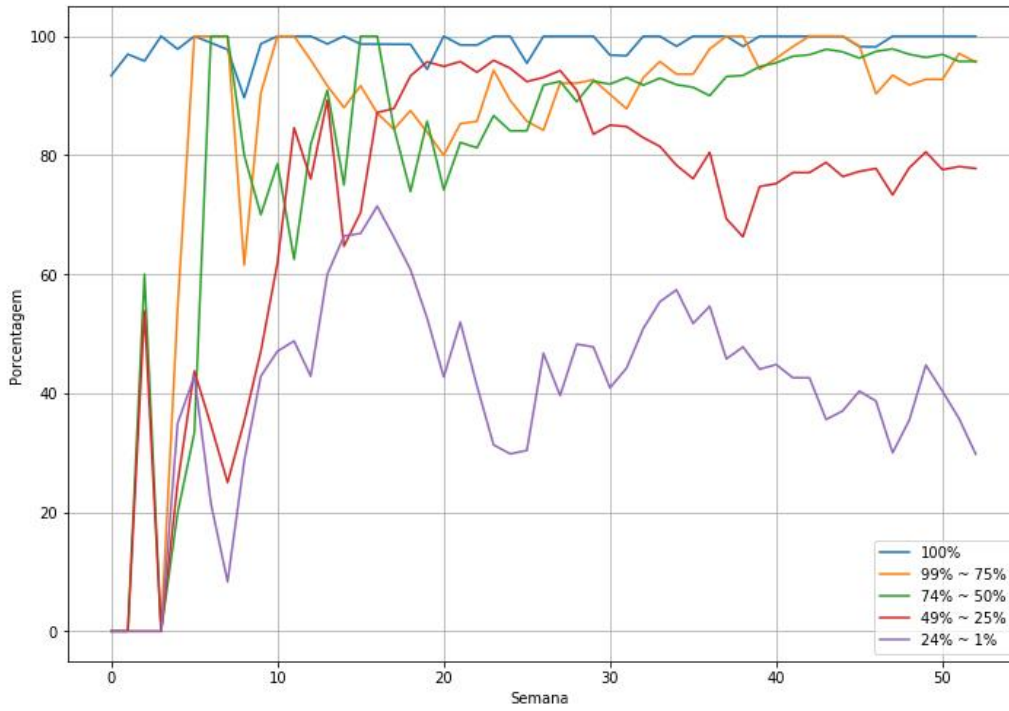
Figura 10: Precisão por setores do atributo critical_rate
