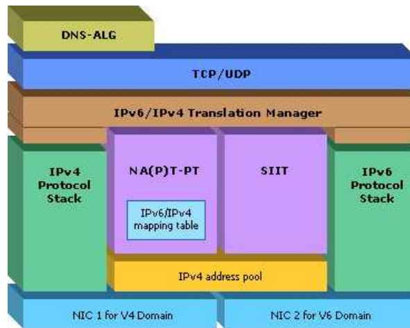
Figura 1: Pilha do Gateway NAT-PT conforme recomendação da RFC2766. [RNP]
