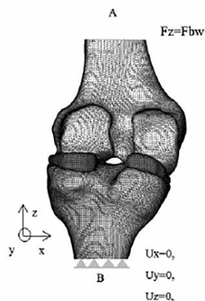
Fig. 2 Modelo computacional, carregamento e constrangimentos (vista posterior).
