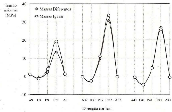
Fig. 8 Tensões máximas na direção inclinada, massas diferenciadas e iguais.
