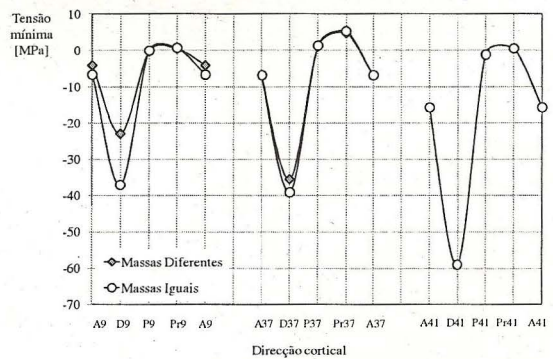
Fig. 10 Tensões mínimas na direção inclinada, massas diferenciadas e iguais.
