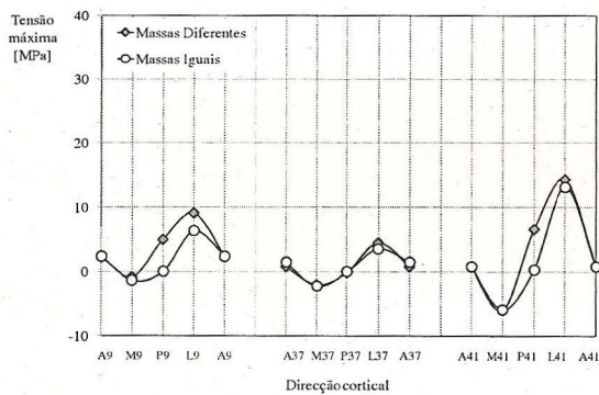
Fig. 7 Tensões máximas na direção horizontal, massas diferenciadas e iguais.
