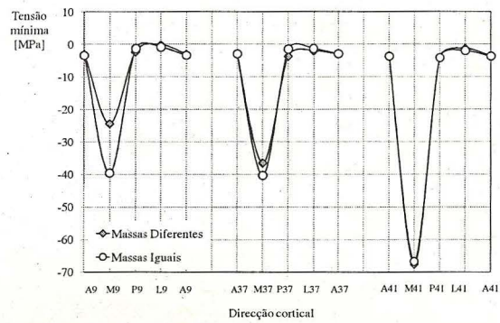
Fig. 9 Tensões mínimas na direção horizontal, massas diferenciadas e iguais.
