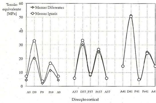
Fig. 6 Tensões equivalentes na direção inclinada, massas diferenciadas e iguais.
