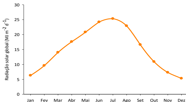
Figura 7 - Radiação solar média (MJ m -2 d -1 ) em Bragança no período 1971-2000
