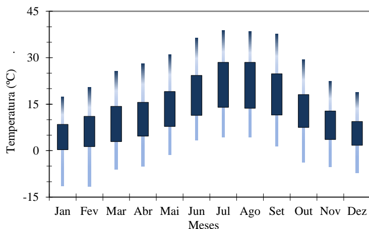
Figura 4 - Amplitude térmica (colunas) e valores absolutos das temperaturas máxima e mínima (extremos da linha vertical) para Bragança, no período 1971-2000.
