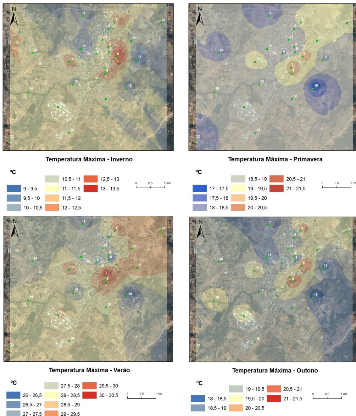
Figura 25 – Isolinhhas das médias das temperaturas máximas diárias, por estações do ano.
