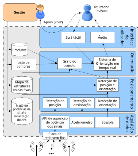
Figura 1 Arquitectura proposta
