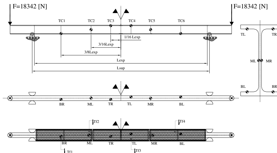
Figura 6 - Caso de estudo e localização dos termopares.
