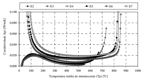
Figura 13 – Variação da condutividade do intumescente com a temperatura.
