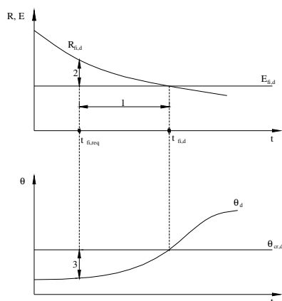
Figura 4 - Domínios de verificação da resistência ao fogo.
