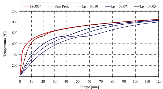
Figura 3 – Análise de um perfil IPE100 protegido com tinta intumescente.
