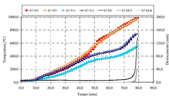
Figura 12 - Resultados dos ensaios E5 a E7.
