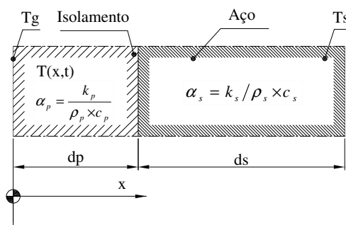
Figura 2 – Modelo unidimensional de transferência de calor.
