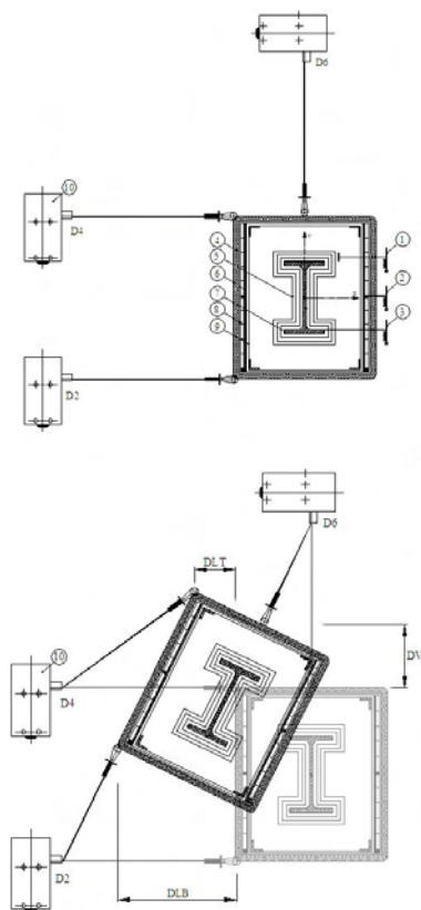
Figura 7 - Esquema do procedimento do ensaio.
