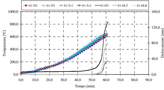
Figura 10 - Resultados do ensaio 1, sem protecção.
