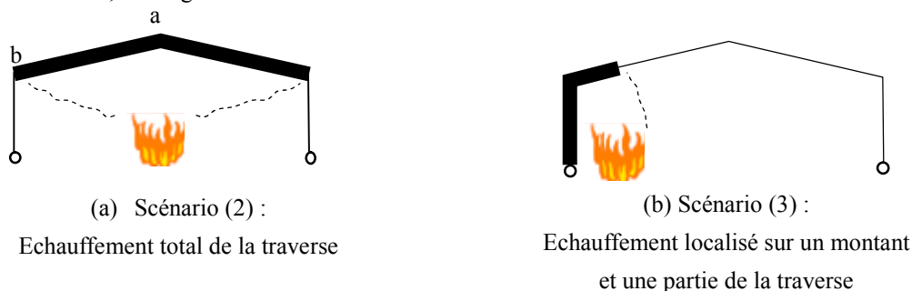
Figure 10 : Profils d'échauffement du modèle pour différents scénarios d'incendie
