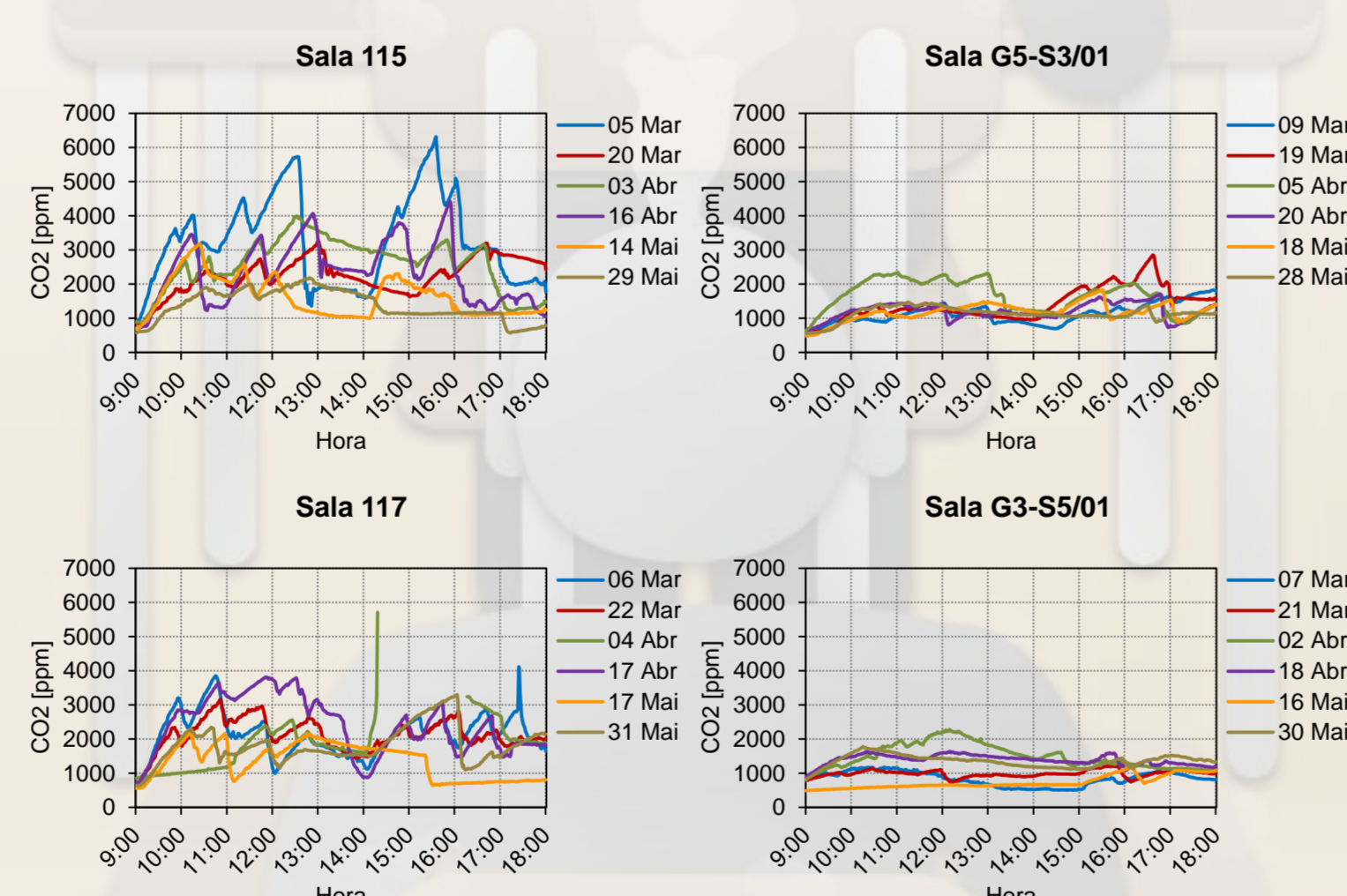
Figura 3 – Concentrações de CO 2 registadas ao longo dos 6 ensaios em cada sala.
