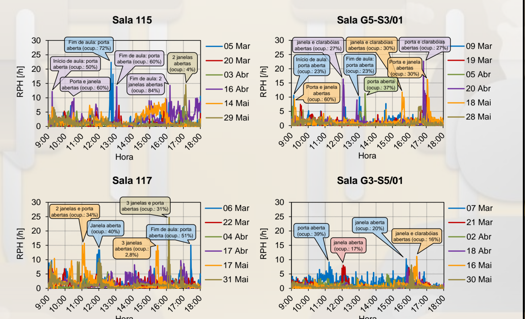
Figura 4 – Renovações de ar por hora com destaques para os valores mais elevados, registadas ao longo dos 6 ensaios em cada sala.
