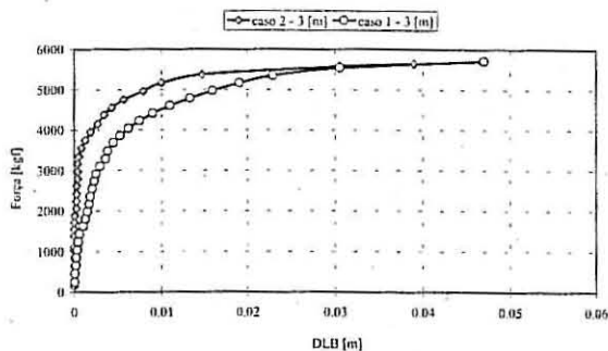
Fig 22 – Deslocamento lateral em baixo (DLB) para ambos os casos.
