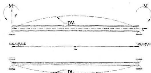
Fig 1 – Geometria e condições de carregamento – caso 1
