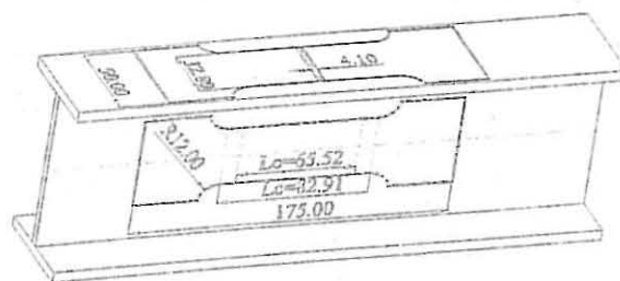
Fig 3 – Dimensões e origem dos provetes
