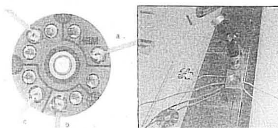
Fig 7 – Roseta de extensómetro e sistema de interferência utilizado.
