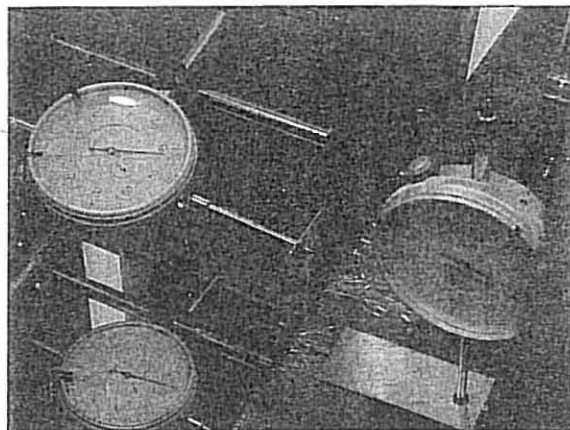
Figura 14 a) – Medição experimental dos deslocamentos DLB, DLC e DV, a meio vão do comprimento da viga.
