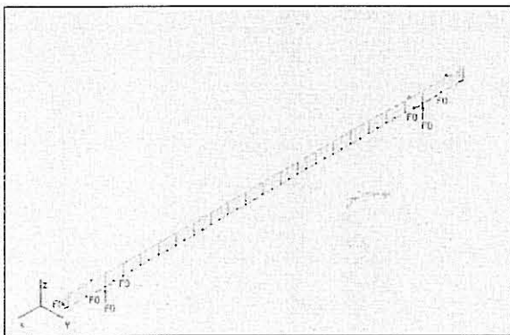
Fig 24 – Modelo de elementos finitos tridimensional, tipo viga, com 22 elementos.
