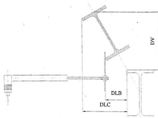
Fig 14 b) – Modelo utilizado para medição deslocamentos DLB, DLC e DV, a meio vão do comprimento da viga.
