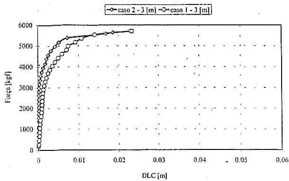
Fig 23 – Deslocamento lateral em cima (DLC) para ambos os casos.
