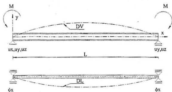
Fig 2 – Geometria e condições de carregamento – caso 2.
