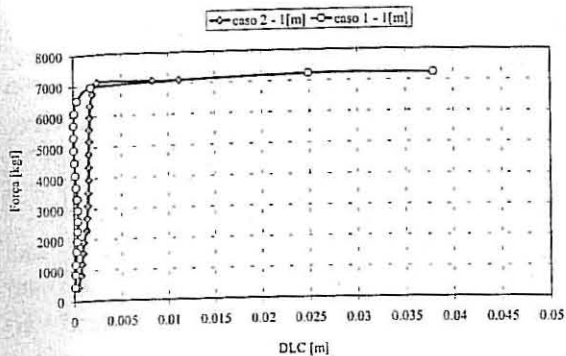
Fig 17 – Deslocamento lateral em cima (DLC) para ambos os casos.
