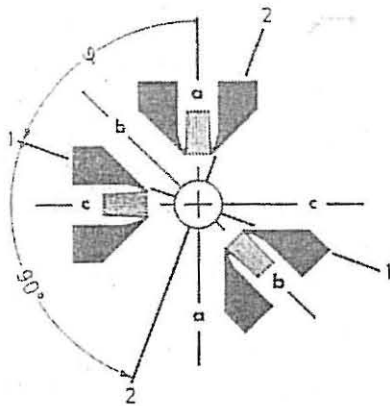
Fig 9 - Direcções principais do estado de tensão residual.
