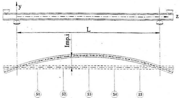
Fig 11 - Controlo da imperfeição geométrica longitudinal dos perfis.
