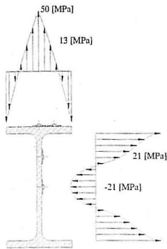
Fig 10 - Distribuição das tensões residuais.
