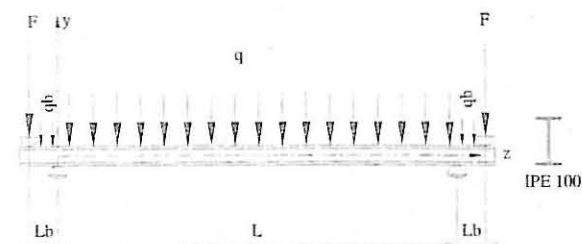
Fig 13 – Sistema de carregamento para viga apoiada com apoios de forquilha.
