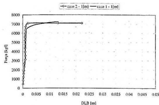
Fig 16 – Deslocamento lateral em baixo (DLB) para ambos os casos.
