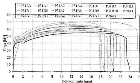
Fig 4 – Resultados de ensaio de tração.
