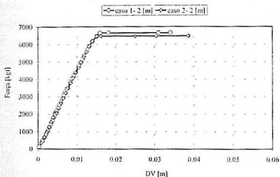
Fig 18 – Deslocamento vertical (DV) para ambos os casos.
