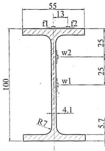
Fig 8 - Posicionamento das rosetas de extensómetros.
