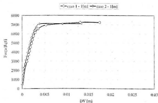
Fig 15 – Deslocamento vertical (DV) para ambos os casos.
