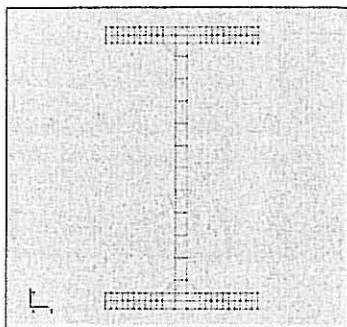
Fig 25 – malha de elementos finitos planos lineares.
