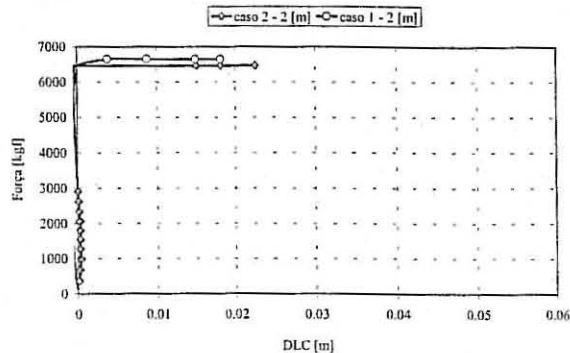
Fig 20 – Deslocamento lateral em cima (DLC) para ambos os casos.
