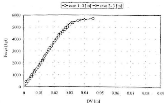
Fig 21 – Deslocamento vertical (DV) para ambos os casos.
