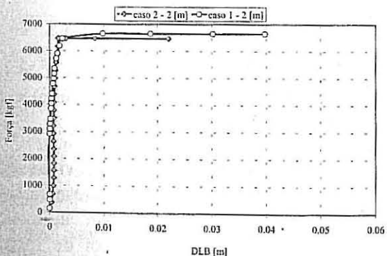
Fig 19 – Deslocamento lateral em baixo (DLB) para ambos os casos.
