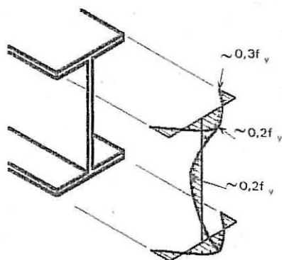
Fig 6 – Distribuição de tensões residuais idealizadas em perfis laminados a quente.
