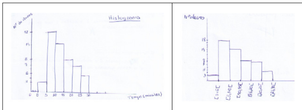
Figura N.º 2 – Dificuldades na construção de histogramas (questionário final)
