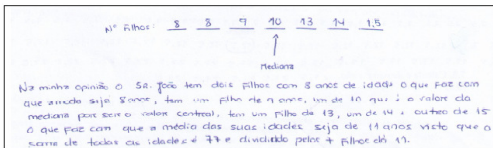
Figura N.º 4 – Exemplo de utilização de alguns critérios (questionário final)
