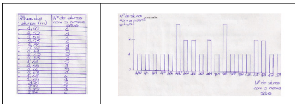
Figura N.º 1 – Tabela de frequências e representação gráfica (questionário inicial)
