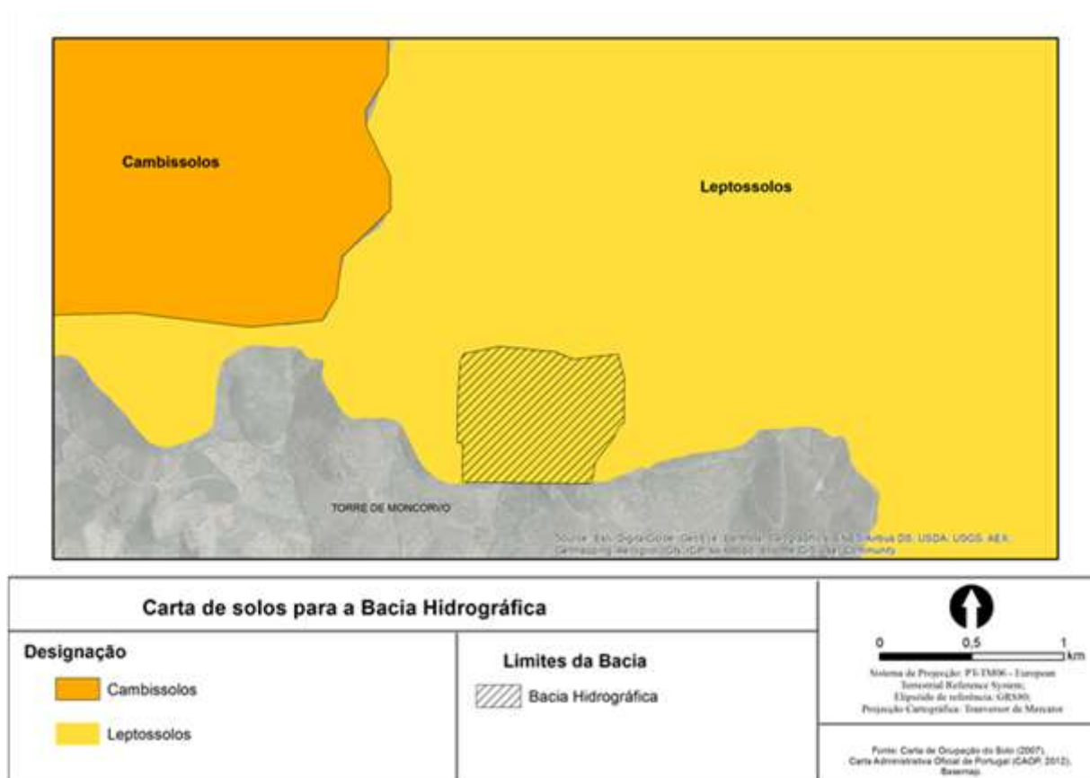
Figura 15- Carta de Solos da bacia hidrográfica.
