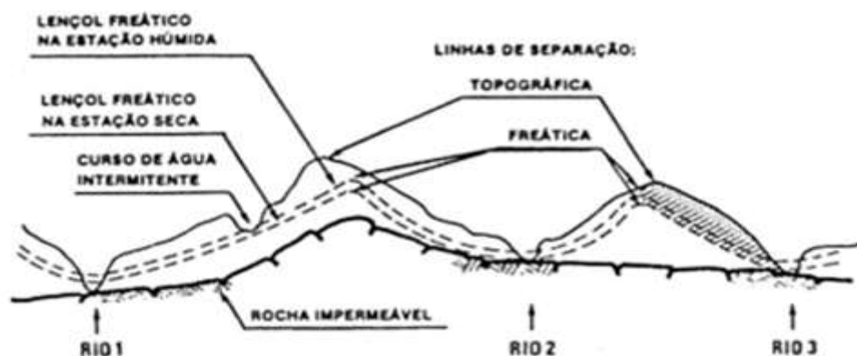
Figura 5- Corte transversal de uma bacia (Lencastre e Franco, 2006).
