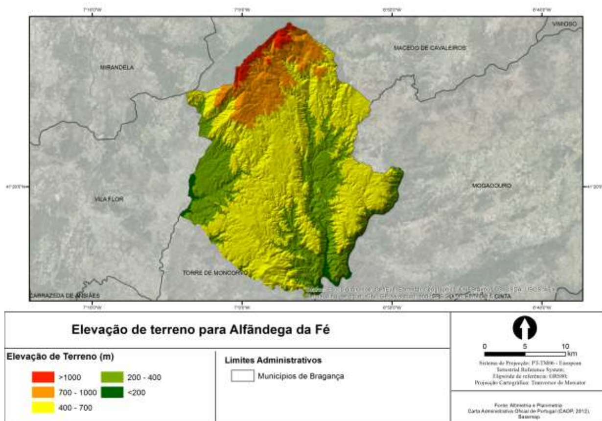
Figura 8- Modelo de Elevação de terreno para Alfândega da Fé.
