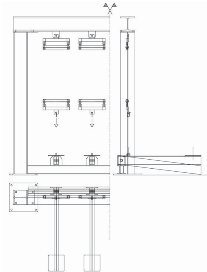
Fig. 8 – Esquema do pórtico concebido para realização de ensaios de fluência e de ruptura em fluência de geossintéticos.
