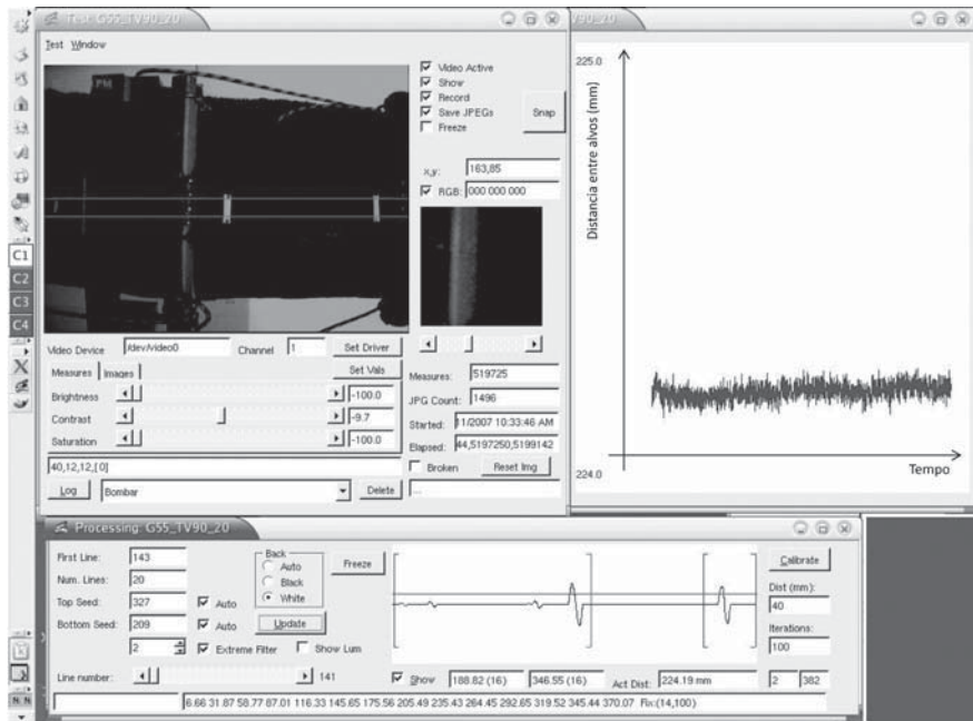
Fig. 15 – Menu de identificação de eventos significativos para o ensaio de fluência ou ruptura em fluência.
