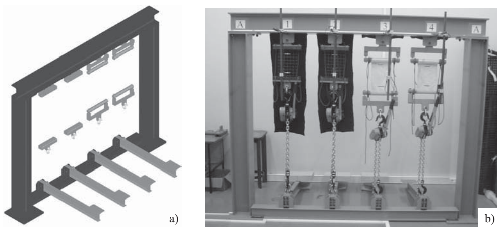
Fig. 9 – Pórtico para realização de ensaios de fluência e de ruptura em fluência de geossintéticos: a) esquema tridimensional; b) vista geral.
