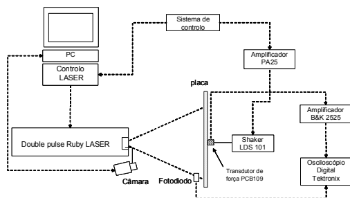
Figura 1 - Esquema da montagem experimental.
