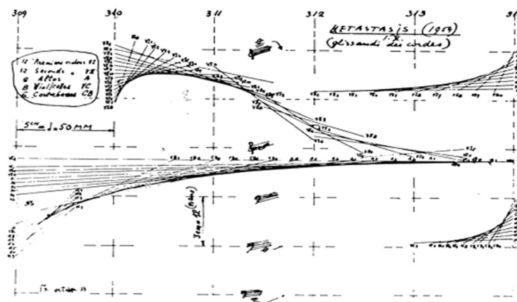
Fig. 6 Metastaseis: compassos 309 a 314 – representação gráfica (XENAKIS, 2012).
