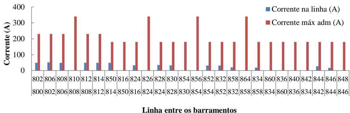
Figura 3.10: Corrente nas linhas com a influência das baterias de condensadores.
