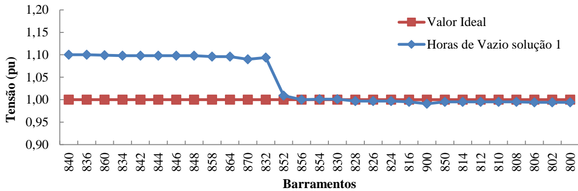
Figura 5.2: Perfil de tensão obtido para a solução 1.
