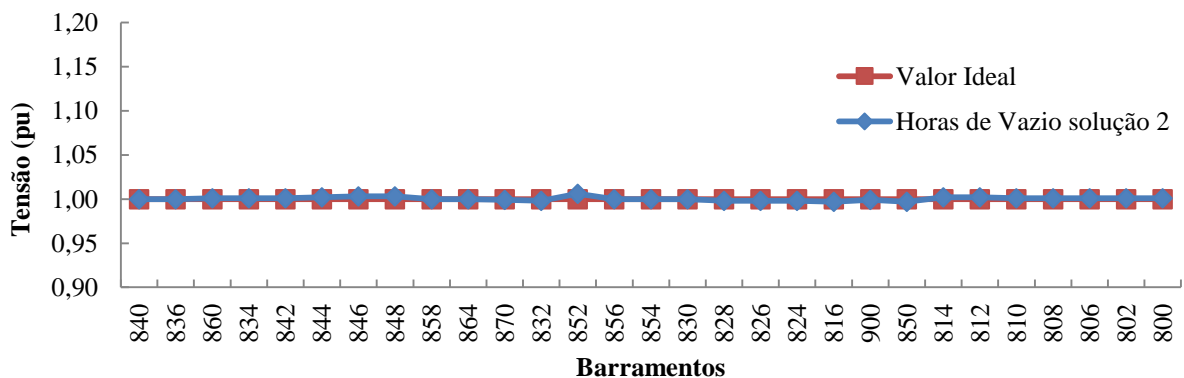
Figura 5.3: Perfil de tensão obtido para a solução 2.
