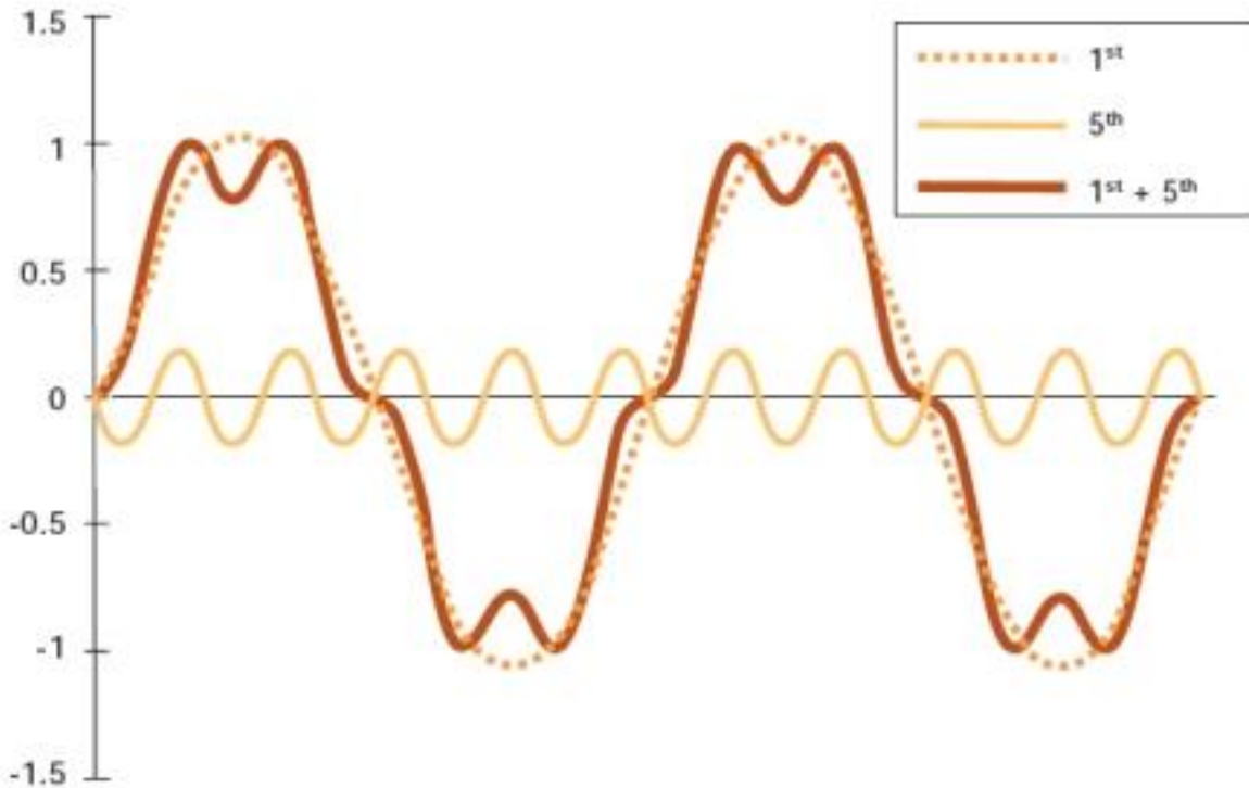
Figura 2.8- Distorsão Harmônica [19].
