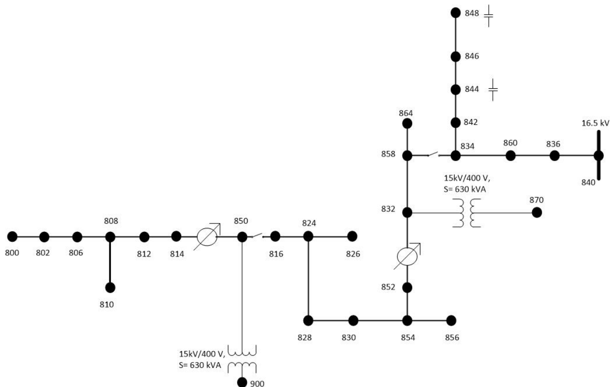
Figura 4.1: Rede com alimentação pelo barramento 840.
