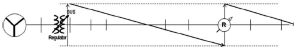
Figura 3.6- Efeito do regulador de tensão nos perfis de tensão [30].
