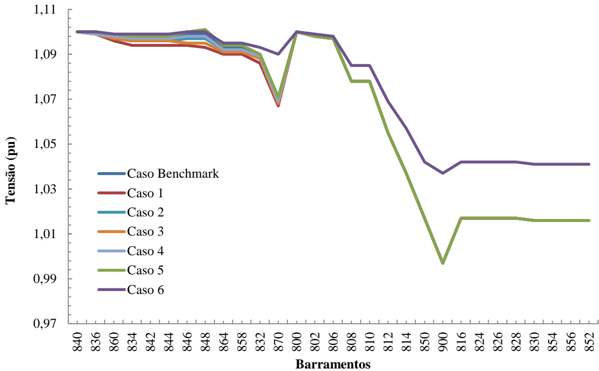
Figura 4.7- Influência das baterias de condensadores nos perfis de tensão.
