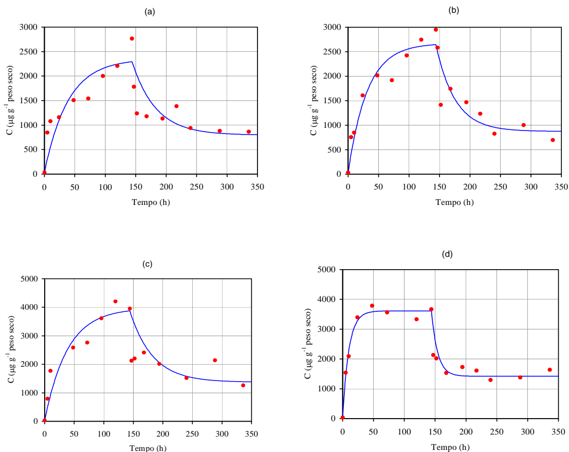
Figura 4: Cinética de acumulação e libertação de cádmio pela Fontinalis antipyretica : efeito da concentração do ião metálico. (a) C_W = 0,64 \text{ mg l}^{-1} , (b) C_W = 0,92 \text{ mg l}^{-1} , (c) C_W = 1,56 \text{ mg l}^{-1} , (d) C_W = 2,26 \text{ mg l}^{-1} ; (— modelo; • dados experimentais).
