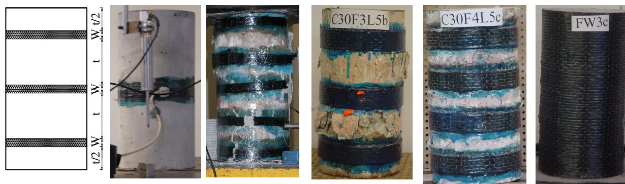
Figura 1 - Esquema de confinamento e fotos de alguns dos sistemas de confinamento adoptados
