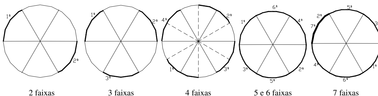
Figura 7 – Disposição do comprimento de entrega das faixas de manta de carbono.
