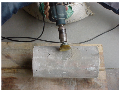
Figura 2 – Esmerilamento do provete nas zonas de fixação das faixas.
