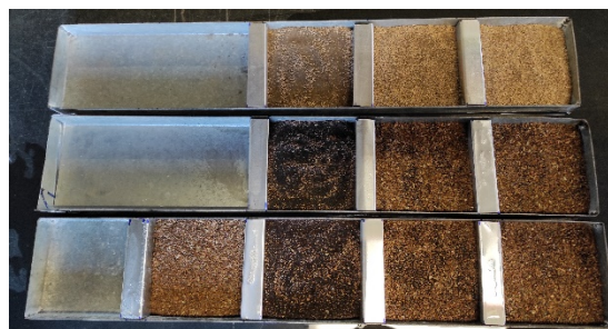
Fig. 1 – Dispositivo experimental para simulação de humedecimento e secagem das amostras.
