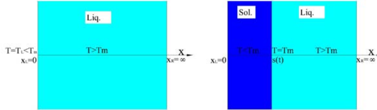
Figura 14 – Modelo unidimensional do problema de Stefan.
