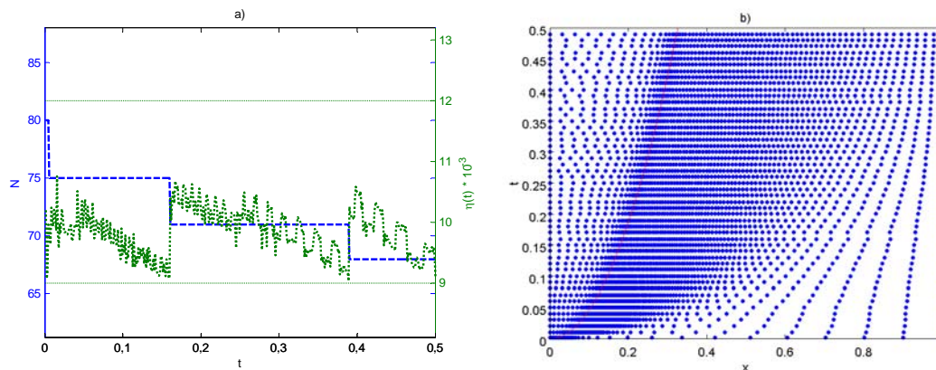
Figura 17 - Resultados da aplicação do método r-h aplicado ao problema de Stefan ( N^0=81 ). a) Evolução do estimador de erro e do número de nós. b) Evolução espacial da malha com o tempo.
