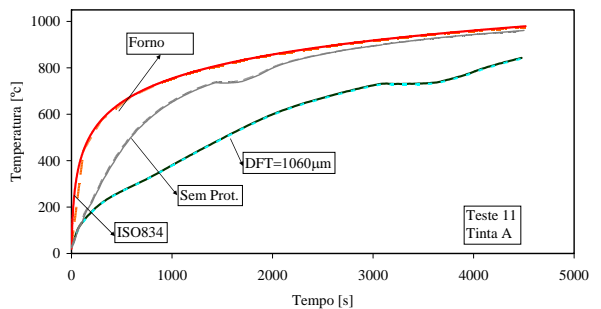
Figura 7 - Variação da temperatura de uma placa de aço com 8 [mm] de espessura e uma espessura de protecção de 1060 [µm] de tinta A.
