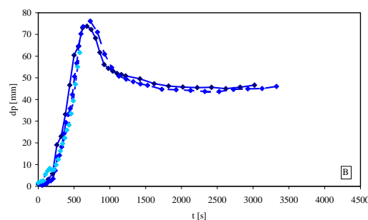
Figura 12 - Resultados experimentais da variação da espessura da camada intumescente dos testes realizados com tinta B.
