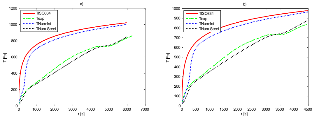
Figura 18 – Comparação dos resultados numéricos e experimentais da evolução da temperatura do aço. a) teste 12. b) teste 11.
