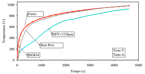
Figura 5 - Variação da temperatura de uma placa de aço com 4 [mm] de espessura e uma espessura de protecção de 1520 [µm] de tinta A.
