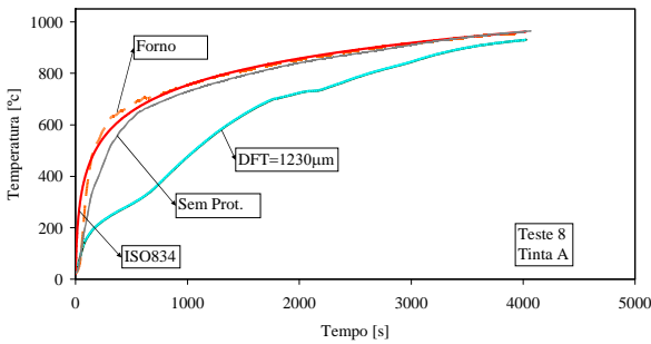
Figura 4 - Variação da temperatura de uma placa de aço com 4 [mm] de espessura e uma espessura de protecção de 1230 [µm] de tinta A.
