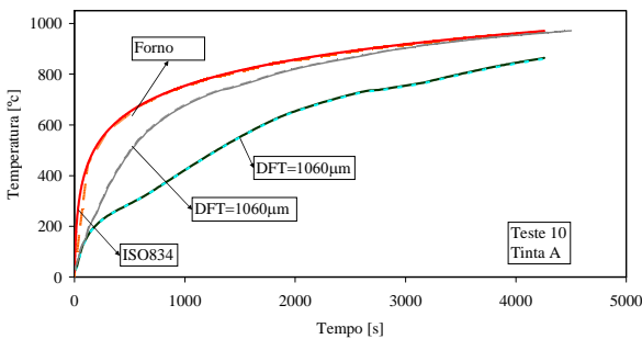
Figura 6 - Variação da temperatura de uma placa de aço com 6 [mm] de espessura e uma espessura de protecção de 1060 [µm] de tinta A.
