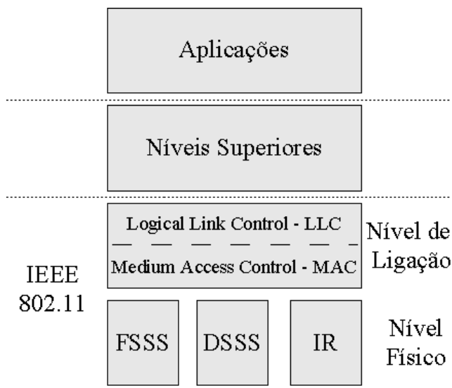
Figura 4 – Arquitectura Protocolar do IEEE 802.11
