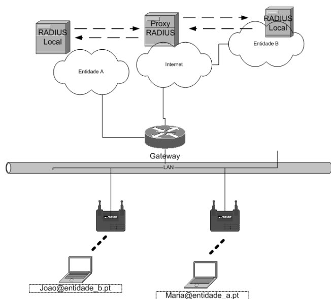
Figura 13 – Utilização de um Proxy RADIUS para suporte de a mobilidade entre redes
