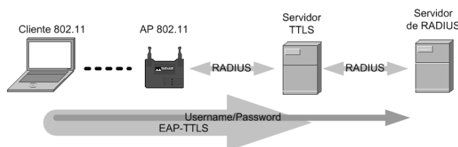
Figura 9 – Princípio de funcionamento do EAP-TTLS
