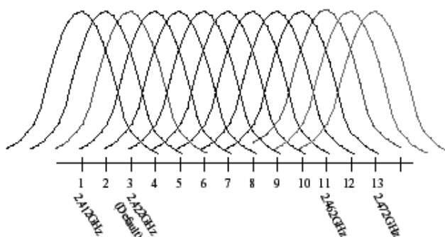
Figura 5 – Gama de frequências e respectivos canais disponíveis numa rede IEEE 802.11b
