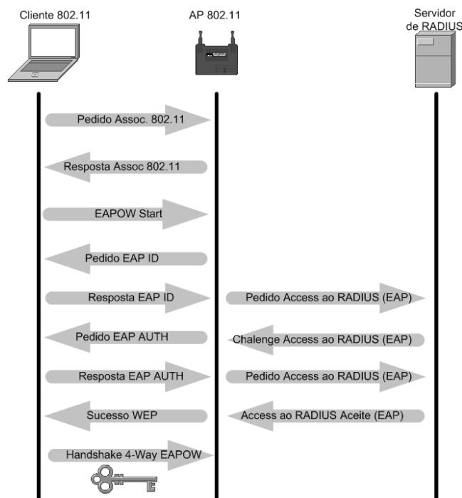
Figura 8 – Processo de autenticação 802.1x
