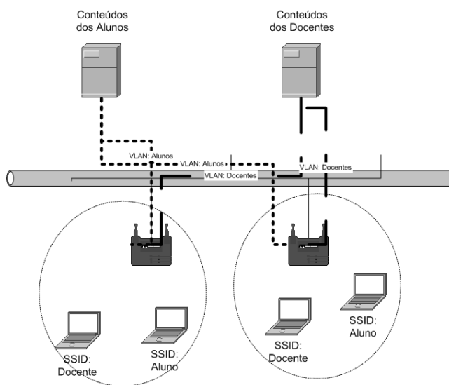
Figura 12 – Mapeamento SSID/VLAN
