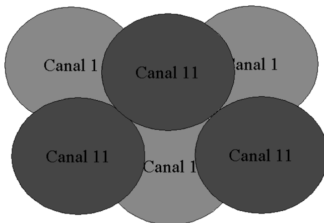
Figura 11 – Disposição de células Wi-Fi com interferências entre os canais
