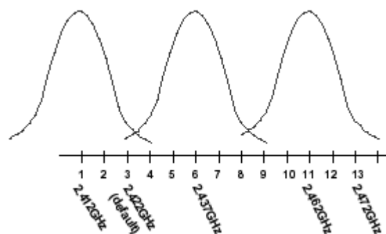
Figura 6 – Canais simultâneos disponíveis numa rede IEEE 802.11b
