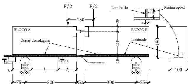
Fig. 12 – Ensaio de arrancamento em flexão com laminados de CFRP.
