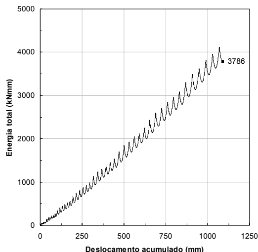
Fig. 7 – Relação energia total vs deslocamento acumulado da gráfico da fig. 8.
