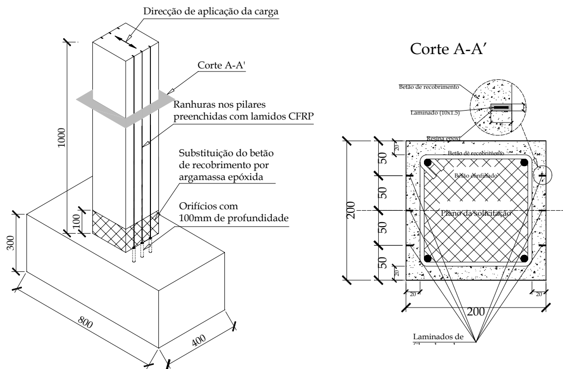
Fig. 3 – Técnica de reforço aplicada.
