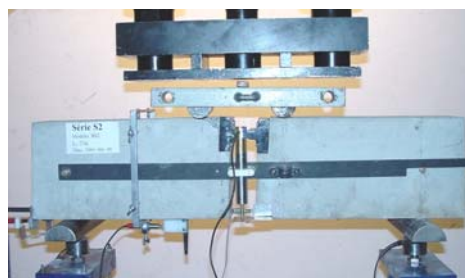
Fig. 13 – Foto do sistema de ensaio.
