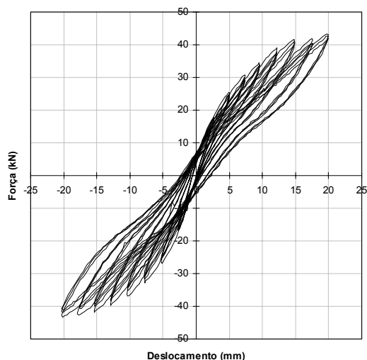
Fig. 6 – Relação força horizontal vs deslocamento correspondente para o pilar P10b_CR.
