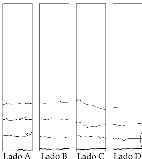
Fig. 10 – Padrão de fendilhação do elemento de pilar P10b_SR.
