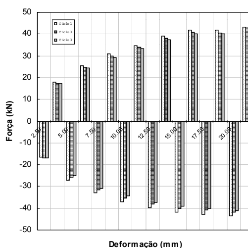
Fig. 9 – Força máxima registada para cada nível de deformação imposto para o P10b_CR.
