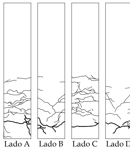
Fig. 11 – Padrão de fendilhação do elemento de pilar P10b_PR.
