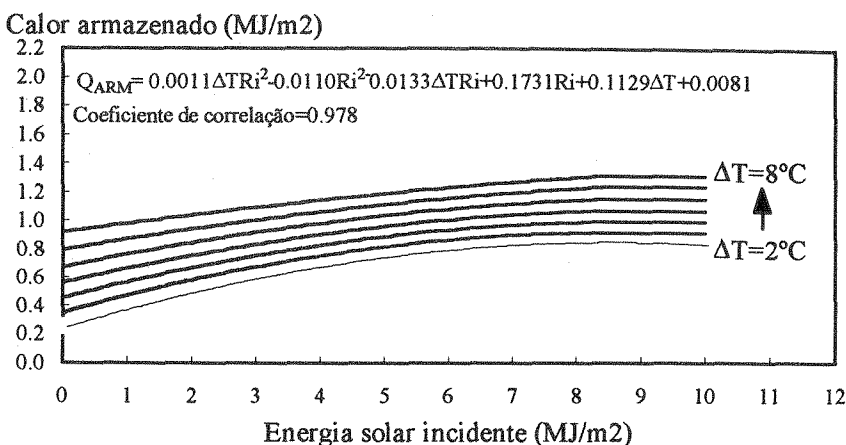
Figura 7 - Calor armazenado por uma parede de tijolo de 11 cm de espessura em função da amplitude térmica diária e da energia solar incidente.
