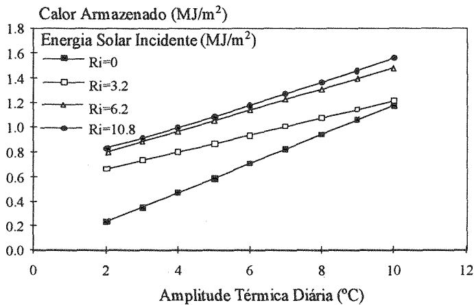
Figura 4 - Variação do calor armazenado com a amplitude térmica diária e com a energia solar incidente para uma parede de tijolo de 11 cm de espessura.
