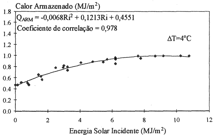
Figura 5 - Variação do calor armazenado com a energia solar incidente, para uma amplitude térmica de 4^\circ\text{C} , para uma parede de tijolo de 11 cm de espessura.
