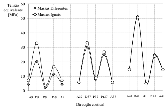
Fig. 6 Tensões equivalentes na direcção inclinada, massas diferenciadas e iguais.
