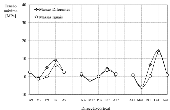
Fig. 7 Tensões máximas na direcção horizontal, massas diferenciadas e iguais.
