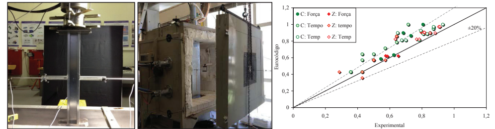
Figura 1 – Setup experimental dos ensaios realizados à temperatura ambiente e ao fogo. Comparação entre os resultados experimentais e os obtidos pelo Eurocódigo 3 da resistência mecânica, tempo e temperatura de resistência ao fogo.
