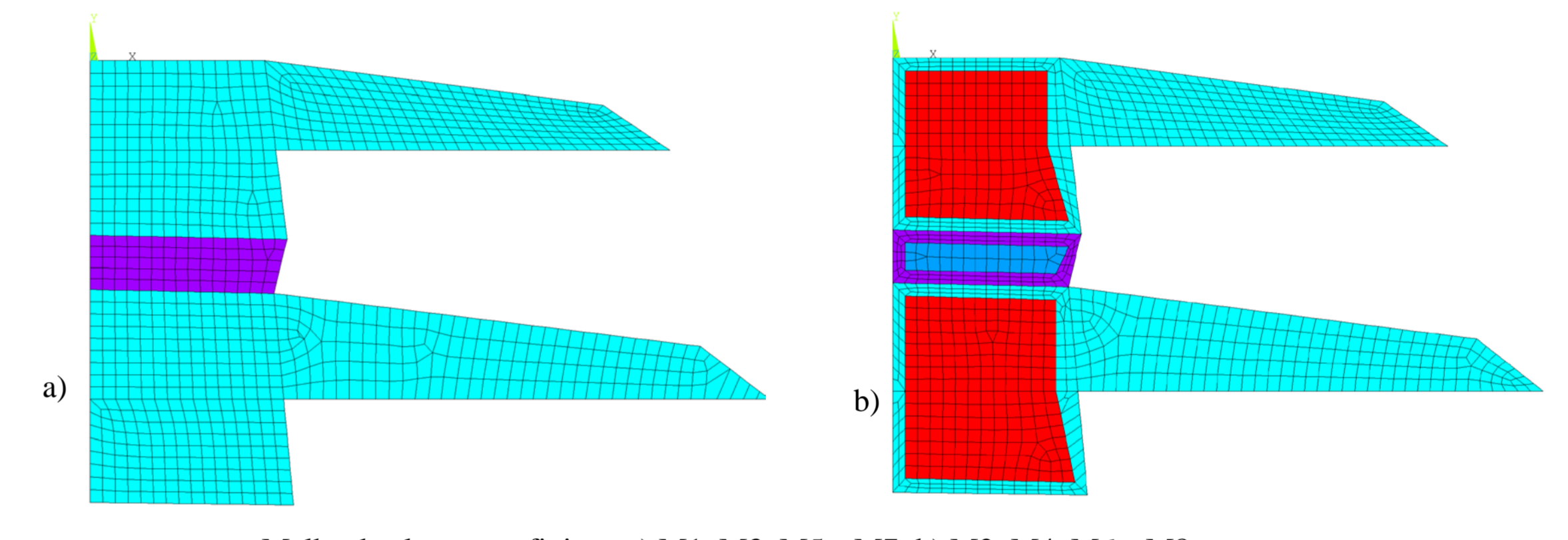
Malha de elementos finitos: a) M1, M3, M5 e M7; b) M2, M4, M6 e M8.
