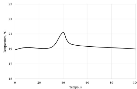
Fig. 8 - Curva de calor da broca para cortical osteoporótico.
