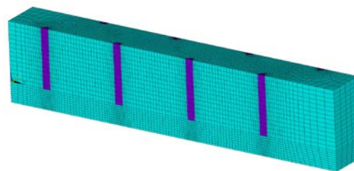
Fig. 6 - Malha de elementos finitos.
