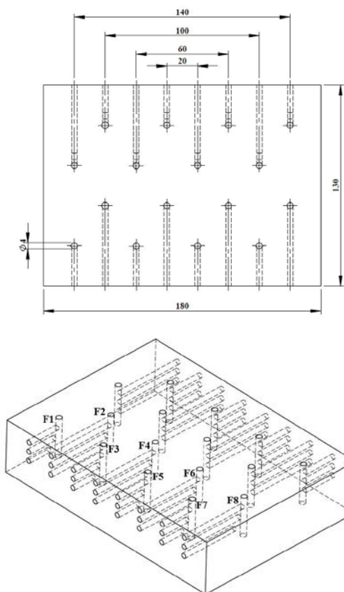
Fig. 5 – Modelo CAD dos blocos em estudo.
