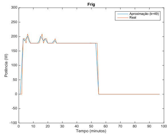
Figura 17: Aproximação ótima característica do Frig por Série de Fourier ( k_{\text{ótimo}}=49 ).
