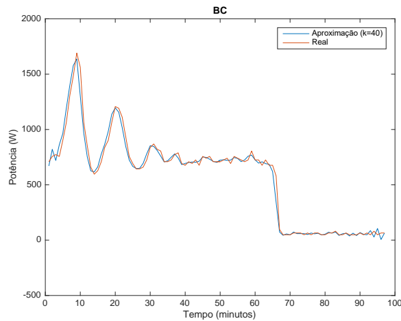
Figura 18: Aproximação óptima característica da BC por Série de Fourier ( k_{ótimo}=40 ).
