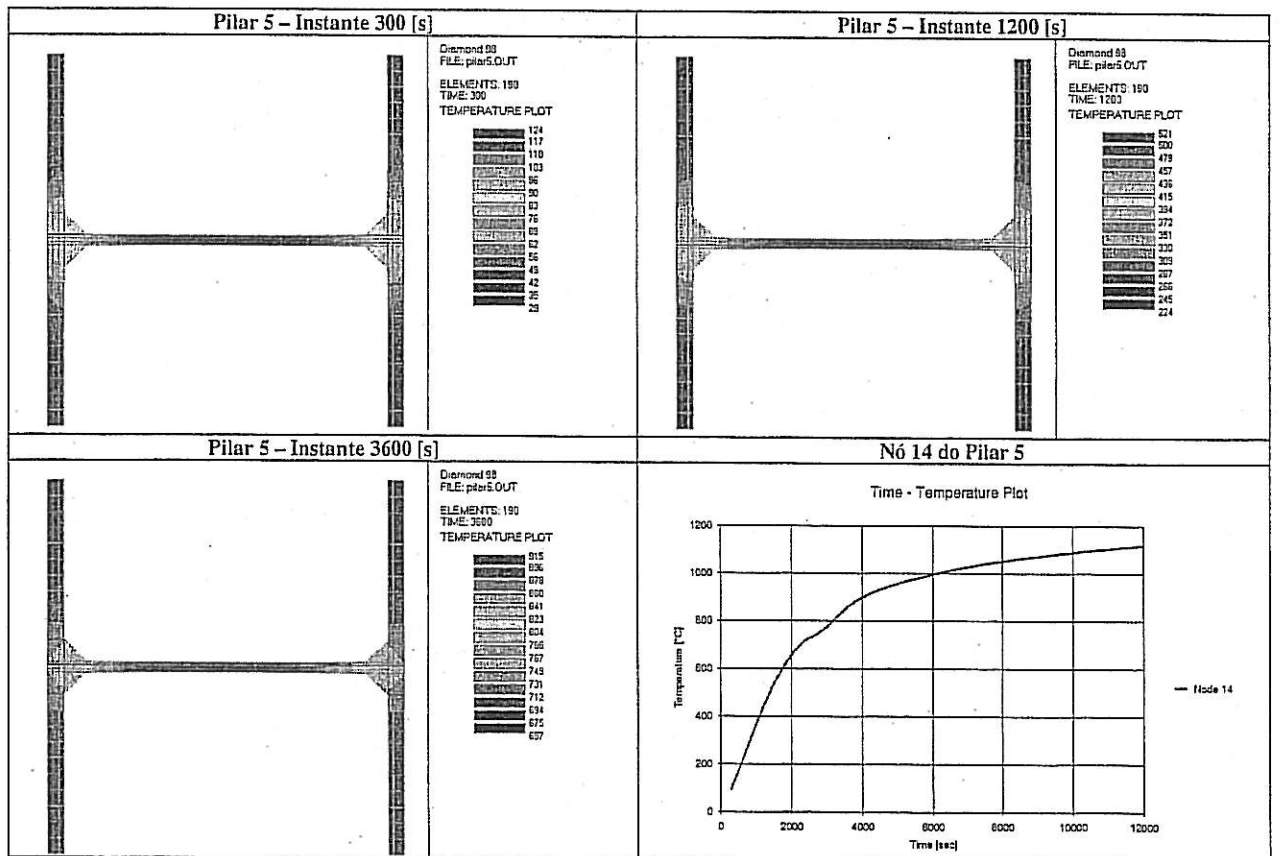
Fig. 9 – Evolução do campo de temperaturas no pilar 5
