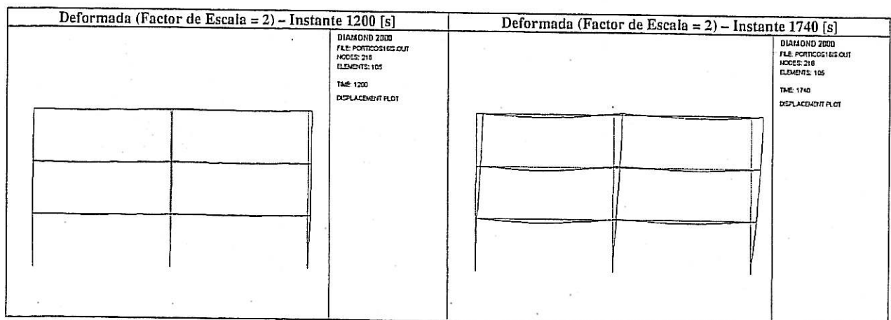
Fig. 18 - Resultados para o cenário de incêndio S6, com isolamento térmico nas vigas
