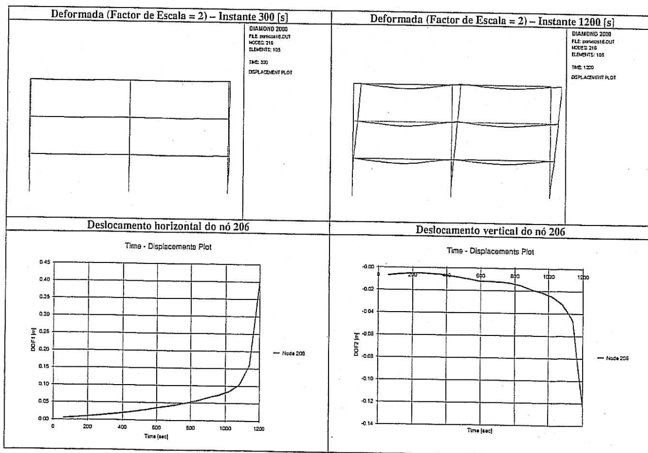
Fig. 13 – Resultados correspondentes ao cenário de incêndio S6
