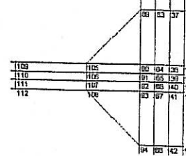
Fig. 7b) - Discretização parcial da secção recta do pilar
