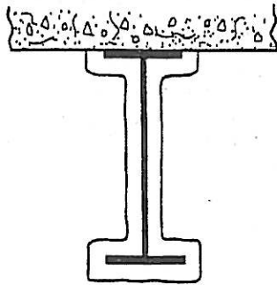
Fig. 16 - Colocação adoptada para a protecção ao fogo
