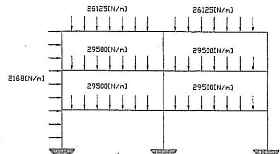
Fig. 3 - Carregamento correspondente à combinação de acções em que o vento é a acção variável dominante
