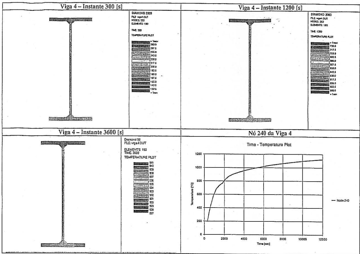
Fig. 10 – Evolução do campo de temperaturas na viga 4
