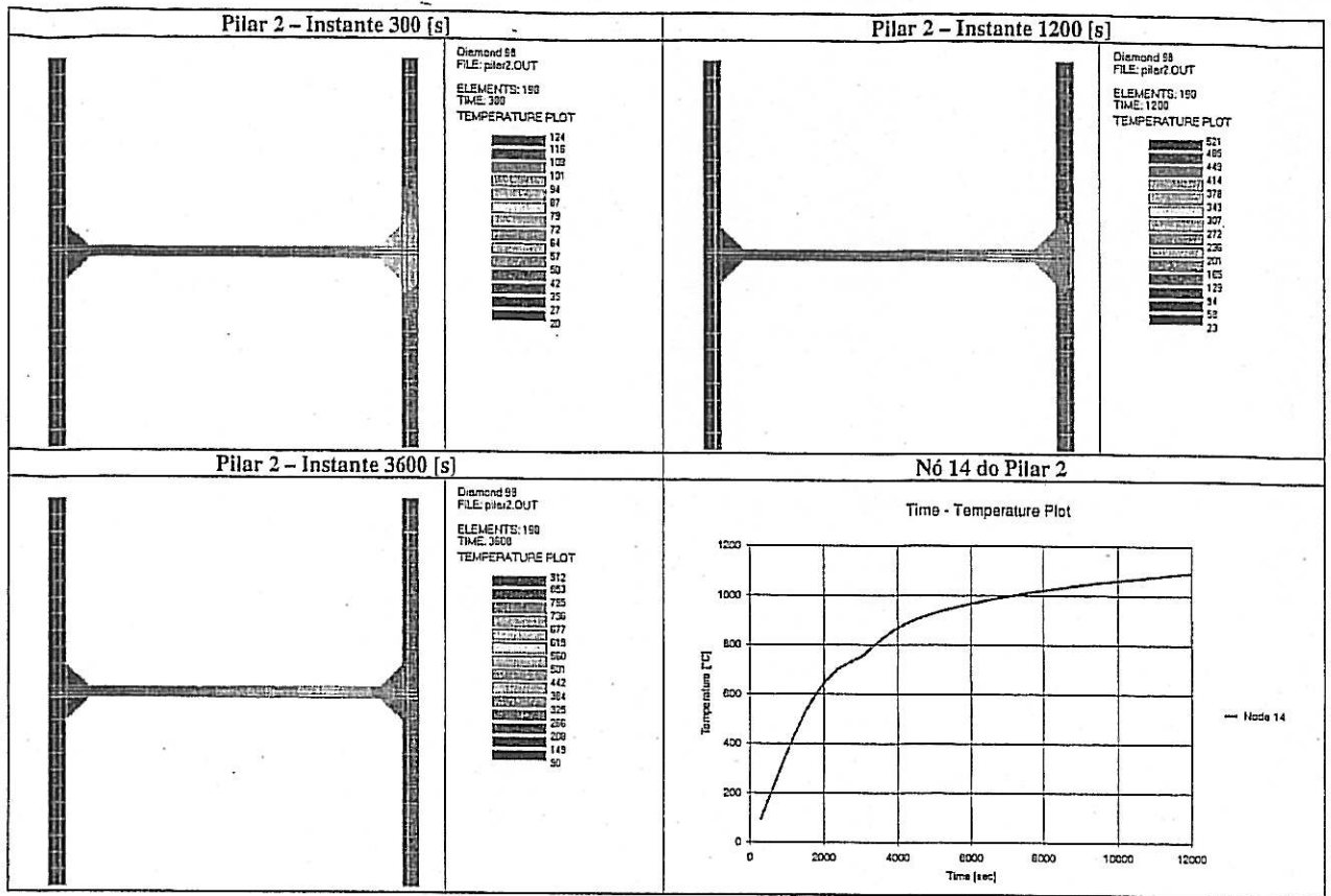
Fig. 8 – Evolução do campo de temperaturas no pilar 2
