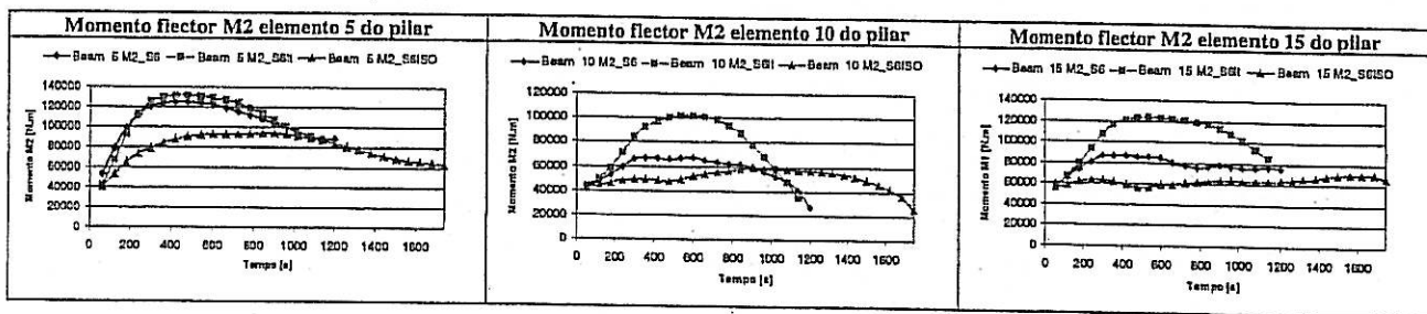
Fig. 20 - Comparação dos momentos flectores nos pilares à esquerda dos compartimentos C1, C3 e C5
