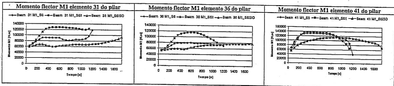
Fig. 21 - Comparação dos momentos flectores nos pilares à direita dos compartimentos C2, C4 e C6
